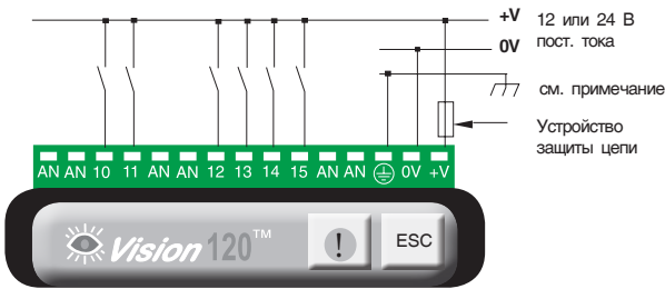
Рис. 3. Дискретные входы
