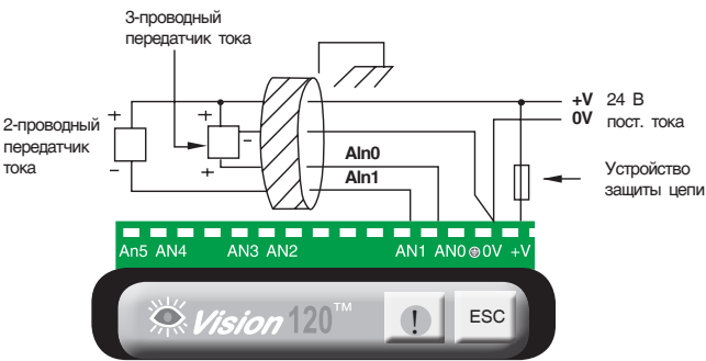
Рис. 2. Аналоговые входы
