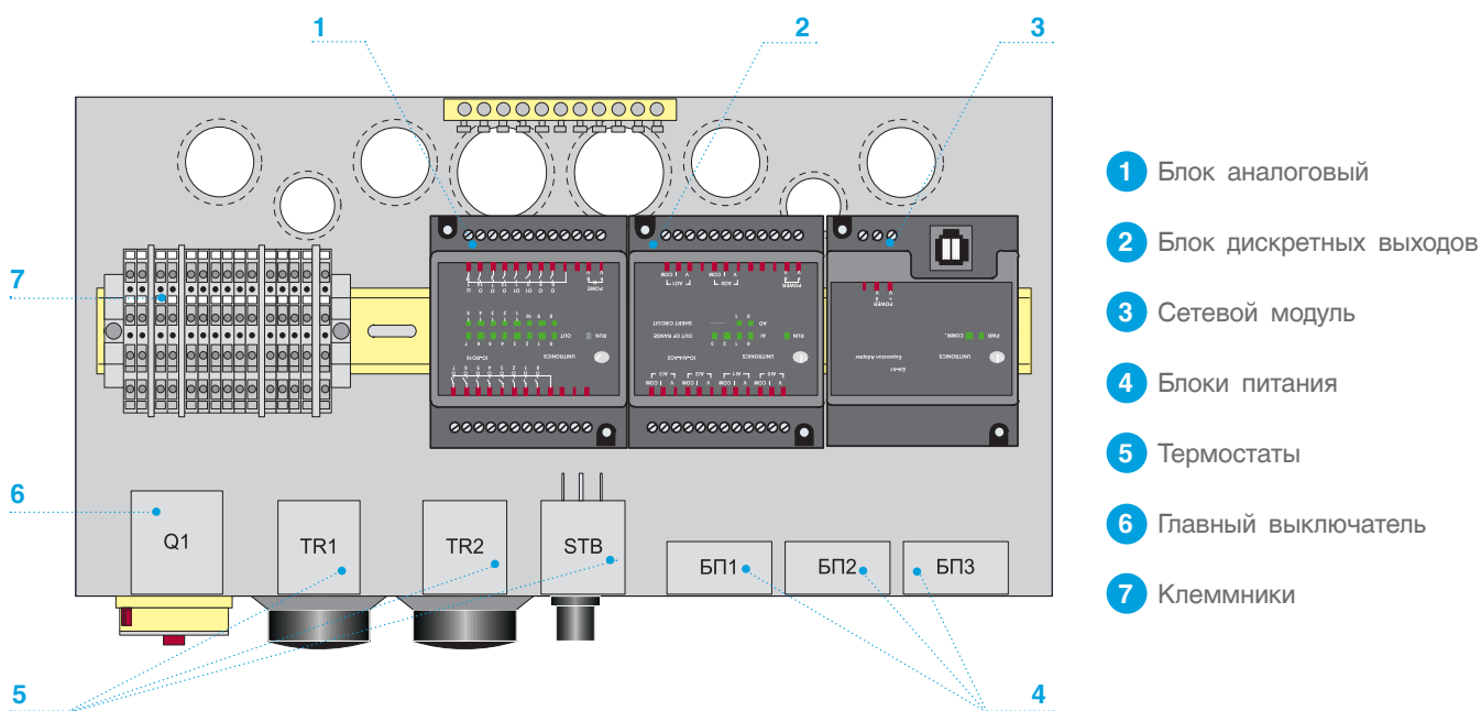
Рис. 17. Расположение элементной базы в блоке «В» (вид сверху)
