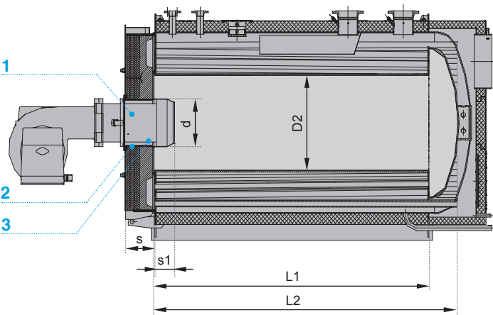
Рис. 5. Установка горелки
