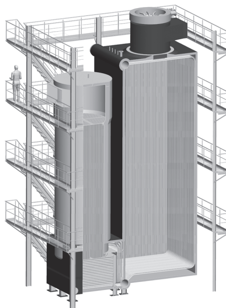
Рис. 2 Общий вид котла ТТ300 с лестницами и площадками обслуживания (*Площадки обслуживания являются дополнительной опцией и заказываются отдельно по запросу)
