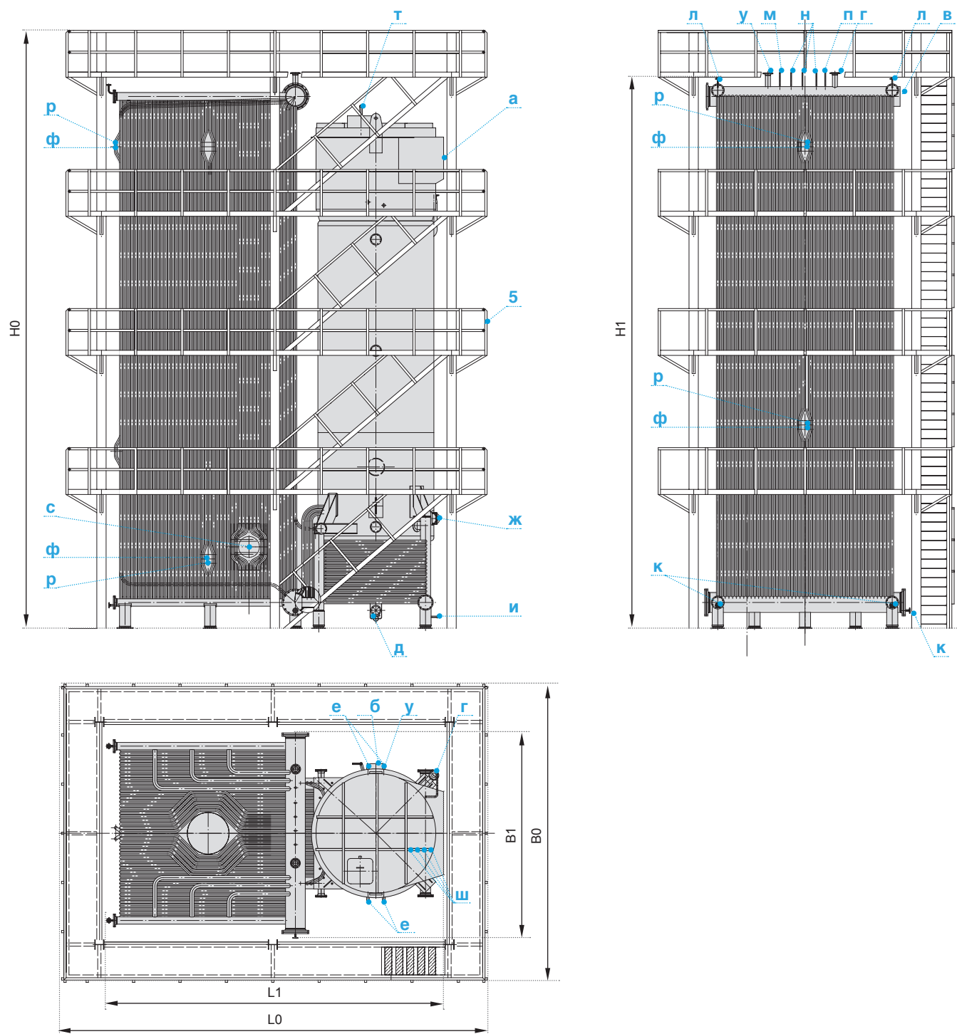
Рис. 5 Основные размеры котлов ТЕРМОТЕХНИК ТТ300
