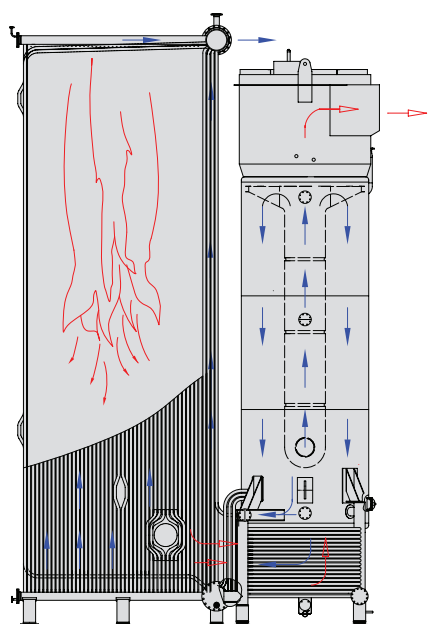
Рис. 4 Принципиальная схема работы котла ТТ300
