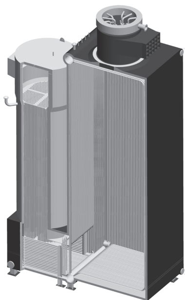
Рис. 1 Общий вид котла ТТ300
