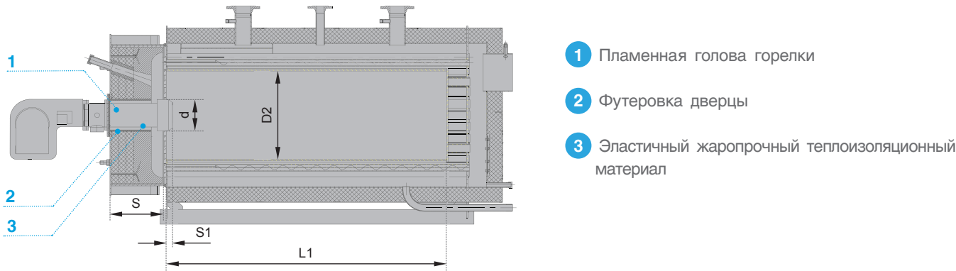
Рис. 5 Установка горелки
