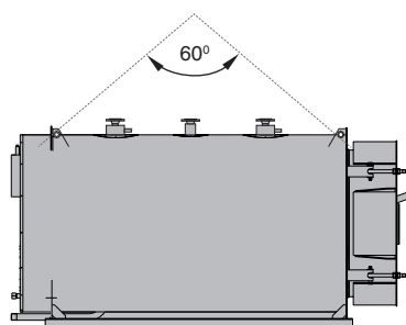
Рис. 7-б Схема строповки котлов теплопроизводительностью 1100 кВт-1740 кВт
