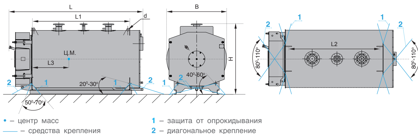
Рис. 6-б – Схема транспортировки котлов теплопроизводительностью 1100 кВт-1740 кВт
