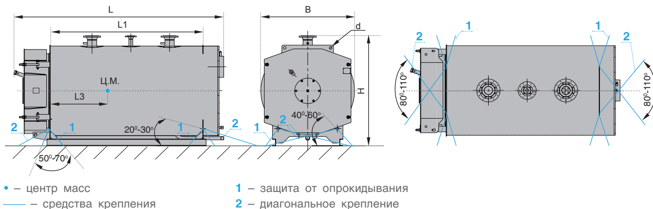
Рис. 6-а – Схема транспортировки котлов теплопроизводительностью 210 кВт-980 кВт
