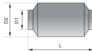
Шумоглушитель дымовых газов (нижний) D1 – внутренний диаметр, D2 – внешний диаметр, L – длина
